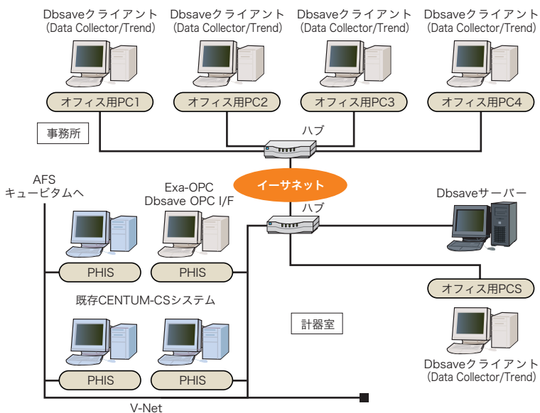
● 横河電機社製CENTUM-CSシステムとの接続例 ●
